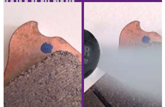
Markierung eines sicherheitsrelevanten Bauteils erlaubt den Nachweis der Originalität (dampfstrahlbeständig, robust)
